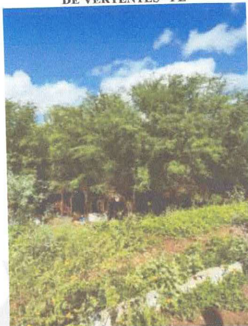
Figura 3. CONSTRUÇÃO DE UM CANAL DE DRENAGEM NO MUNICÍPIO DE VERTENTES - PE
